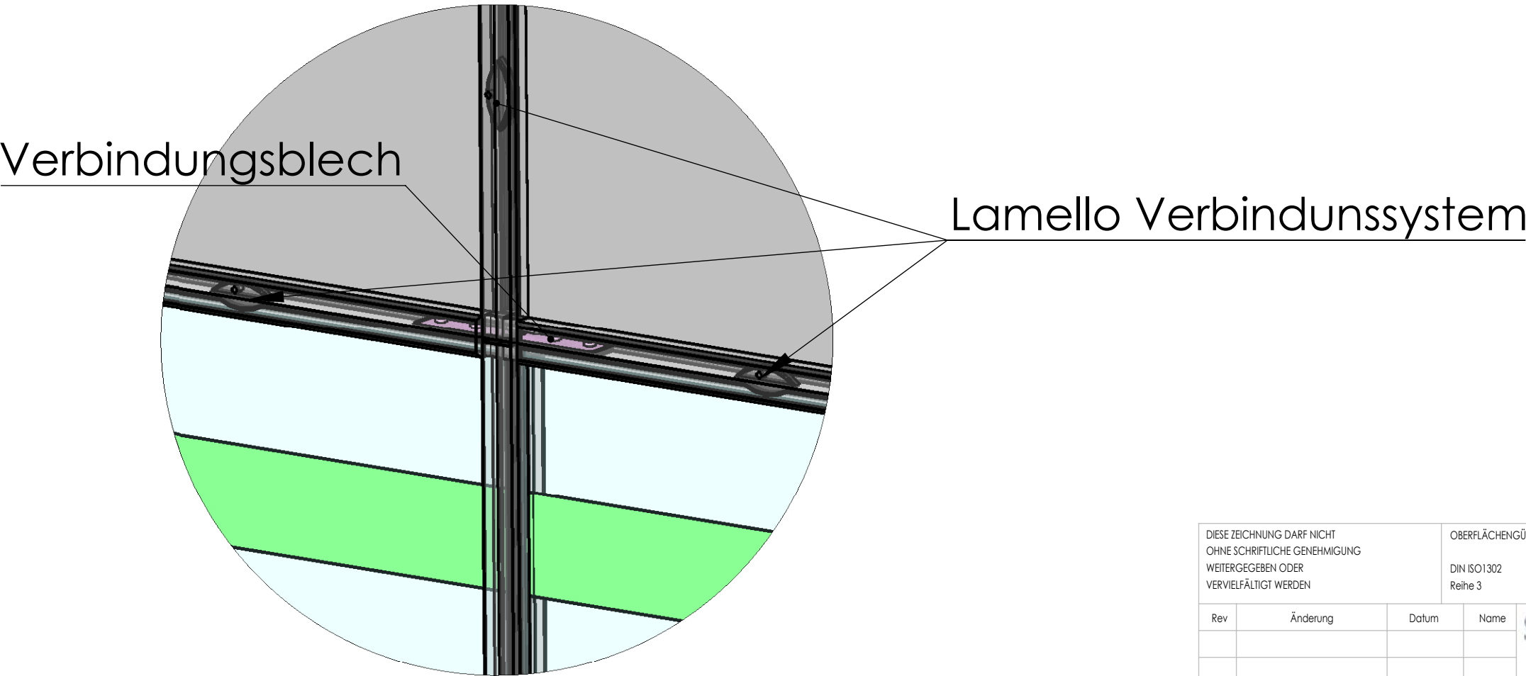
DETAIL J MAßSTAB 1 : 5
